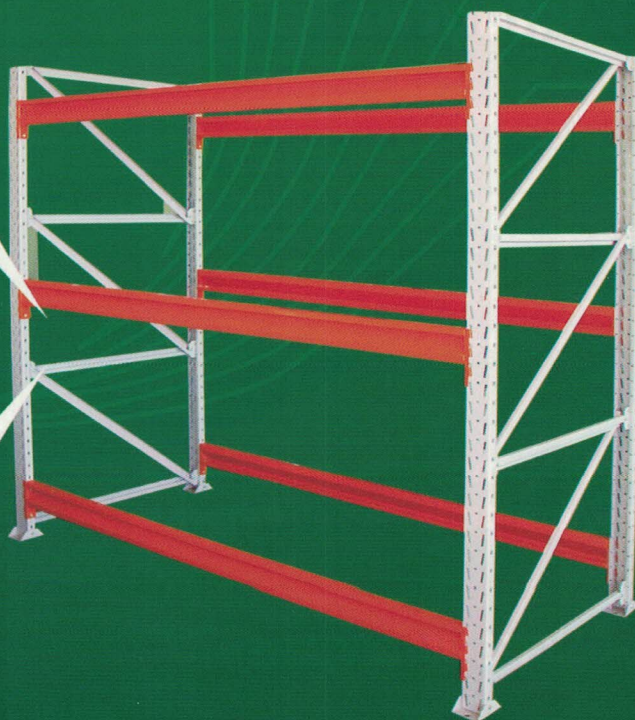
PPM - Estrutura de aço parafusada com compensado Medidas: 2 x 1,10 x 0,50m
