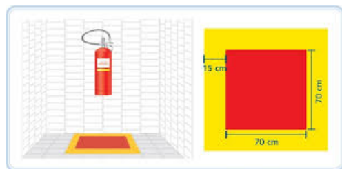
Figura 3.3: Marcação no piso das instalações industriais
